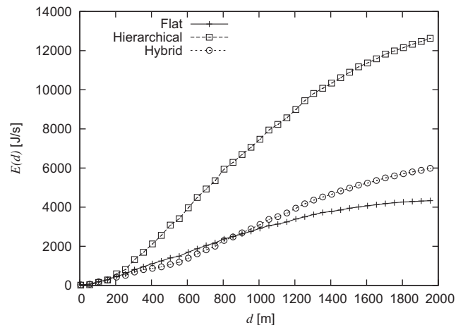
(d) Energy consumption in network.
